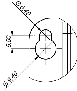
DETAY B ÖLÇEK 1 : 1
