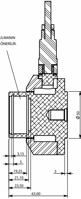
KESİT A-A
