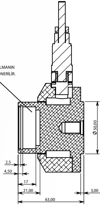
KESİT A-A
