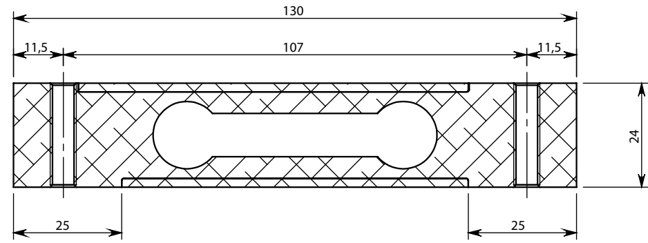
KESIT A-A
