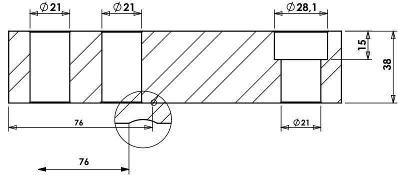
KESİT A-A ÖLÇEK 1 : 2
