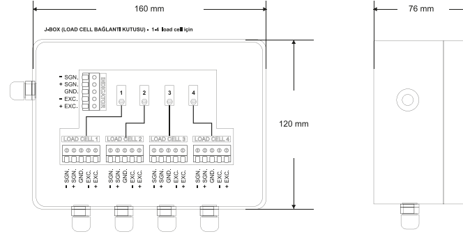
1-4 lü j box ölçüler ve bağlantı şeması
