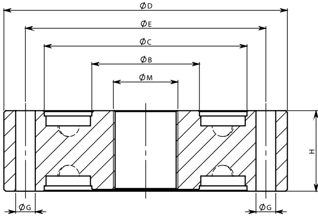
KESİT A-A
